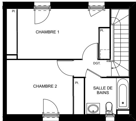
ÉTAGE - BASE
